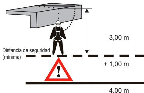
16 Caída lateral sobre el borde
