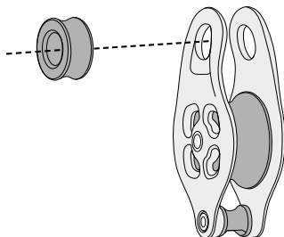
Pinto Rig 2: PUL141 Pinto Rig Spacer: PUL120-SPA
